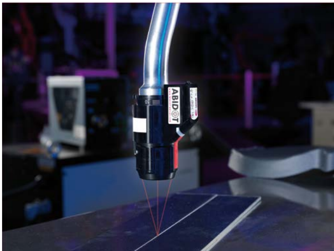
Kuva 3.: ABIDOT-ohjelmointiavustin
